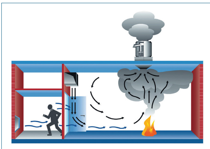
Bild 9: Abschirmung der Brandraumentür durch ebene Luftschleier
