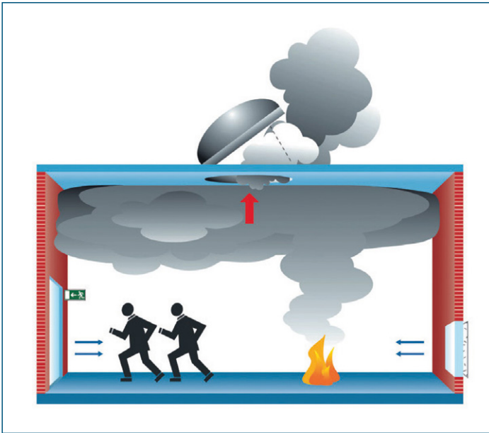
Bild 5: Schichtung bei Einsatz von natürlichen Rauchabzugsanlagen (NRA) Quelle: TROX GmbH
